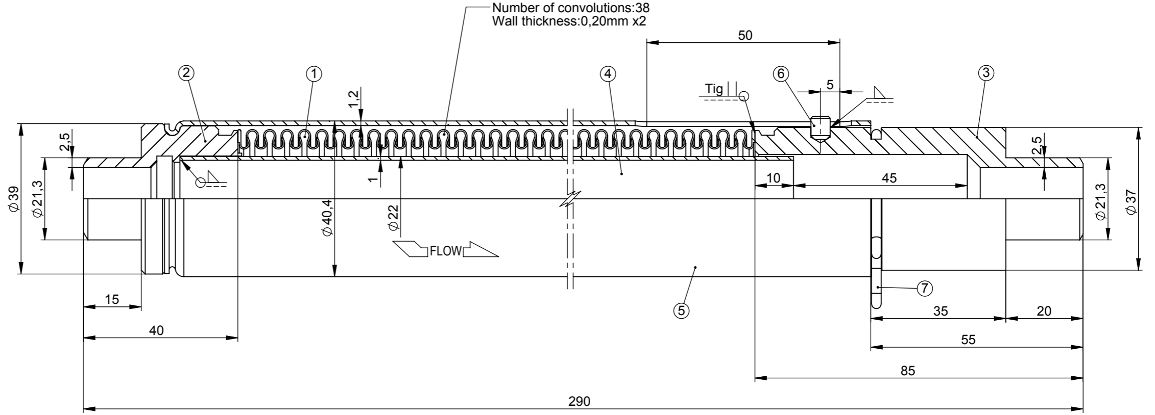
SECTION A-A
